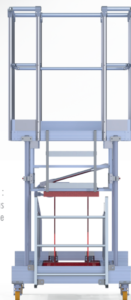
Vue de face : le châssis ne dépasse pas la plateforme
