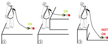
Klareringshøyden under brukerens føtter skal være minst* :
