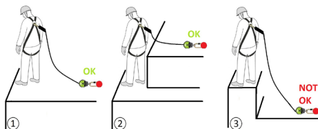
Il tirante d'aria deve essere ad almeno*:
