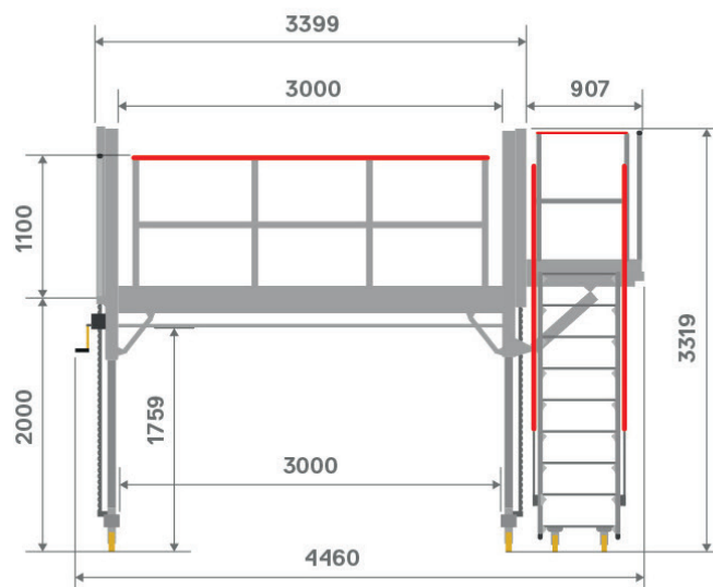
Accès par escalier à 4 montants à palier
