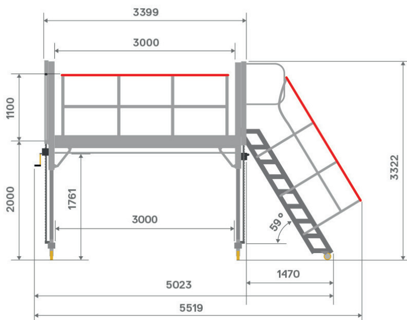
Accès par escalier à 4 montants
