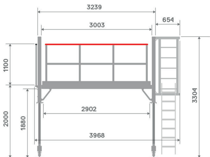
Accès avec échelle
